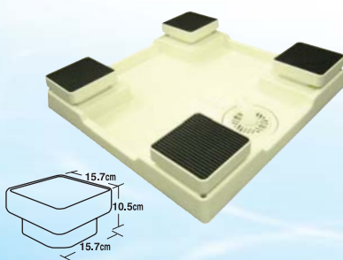
イージースタンド (テクノテック社製) PP樹脂・防振ゴムシート貼り(上面のみ)
